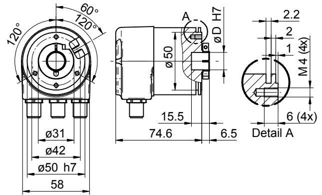
BMSH/BMMH 58 flexible, IP 67
